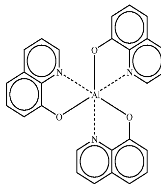
Alq 3
